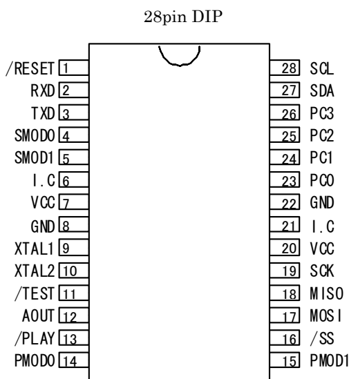
図 3.1 ピン配置(Top View)
