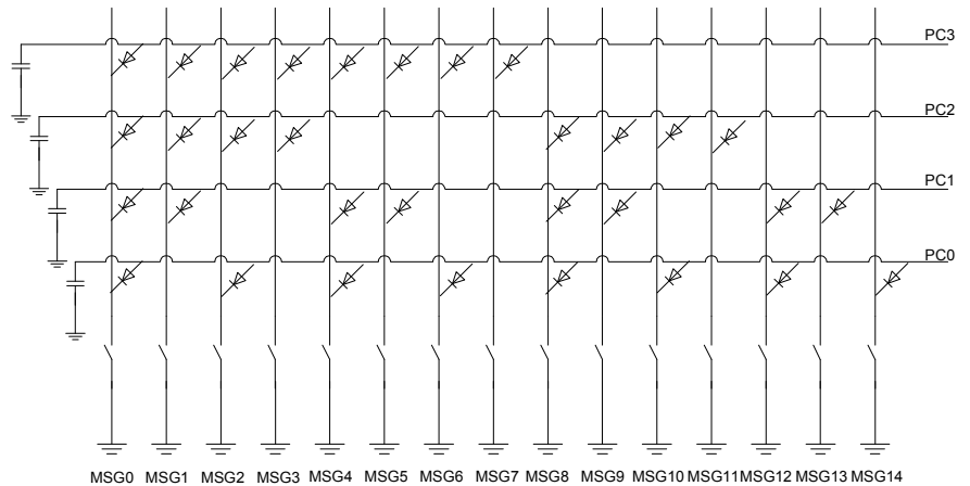
図9.1 スタンドアロンモード(プリセットメッセージ)回路例
